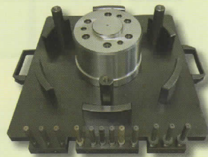
汽車零件孔位檢具
