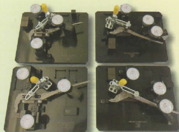
手工具附表量具
