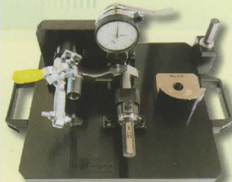
孔位·圓弧位置度附表量具
