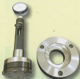
特殊溝內徑比測附表量具
