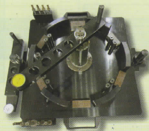
汽車零件孔位附表量具
