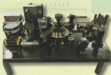
汽車零件孔位綜合檢具
