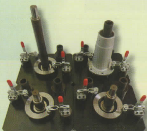
孔位與同軸度檢具
