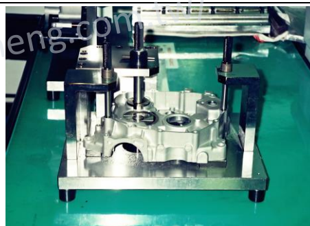
右箱体外廓孔位检具
