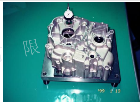
左箱体轴孔孔距检具
