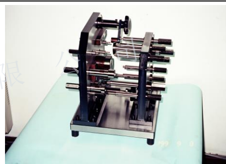
左、右箱体孔位检具
