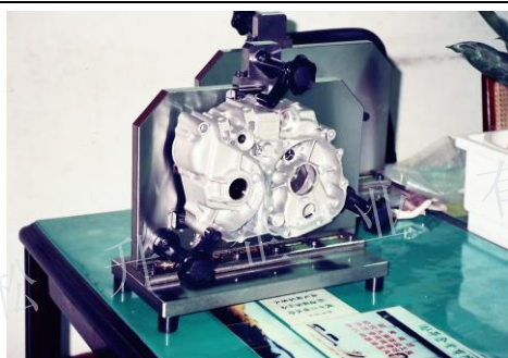
左、右箱体内腔孔位检具
