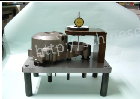
左箱盖孔位检具
