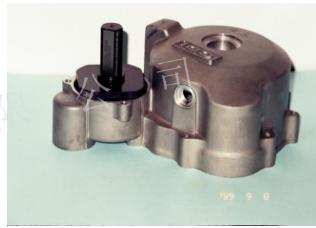
左箱盖孔径同轴度检具
