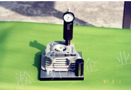
汽缸头孔深度检具
