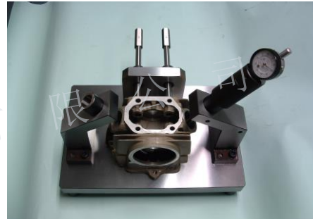
汽缸头孔位及端面距深度检具
