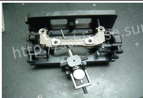
支架圆弧附表检具
