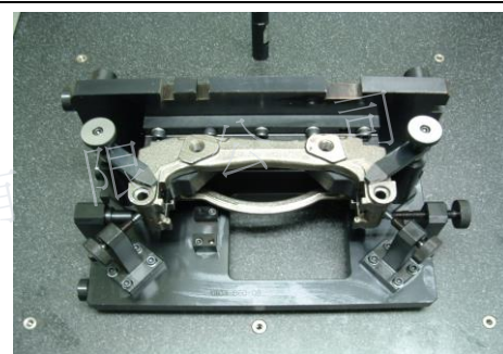
支架位置比测检具
