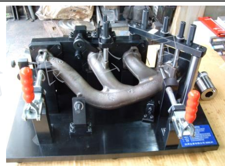
排气管孔位.位置检具
