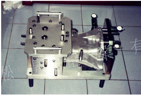
引擎油底壳综合量具
