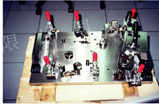
引擎 COVER 孔位检具
